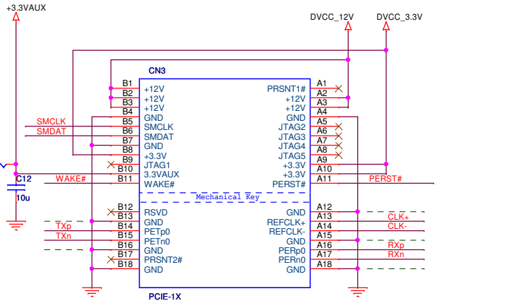
PCI-E 1x Slot
