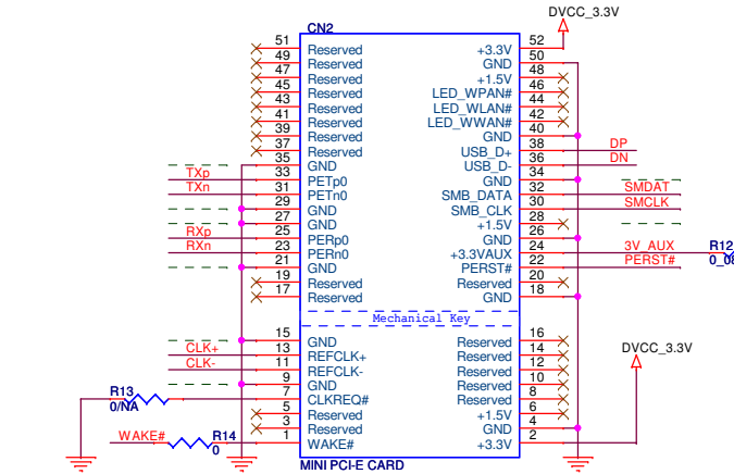
Mini PCI-E Card
